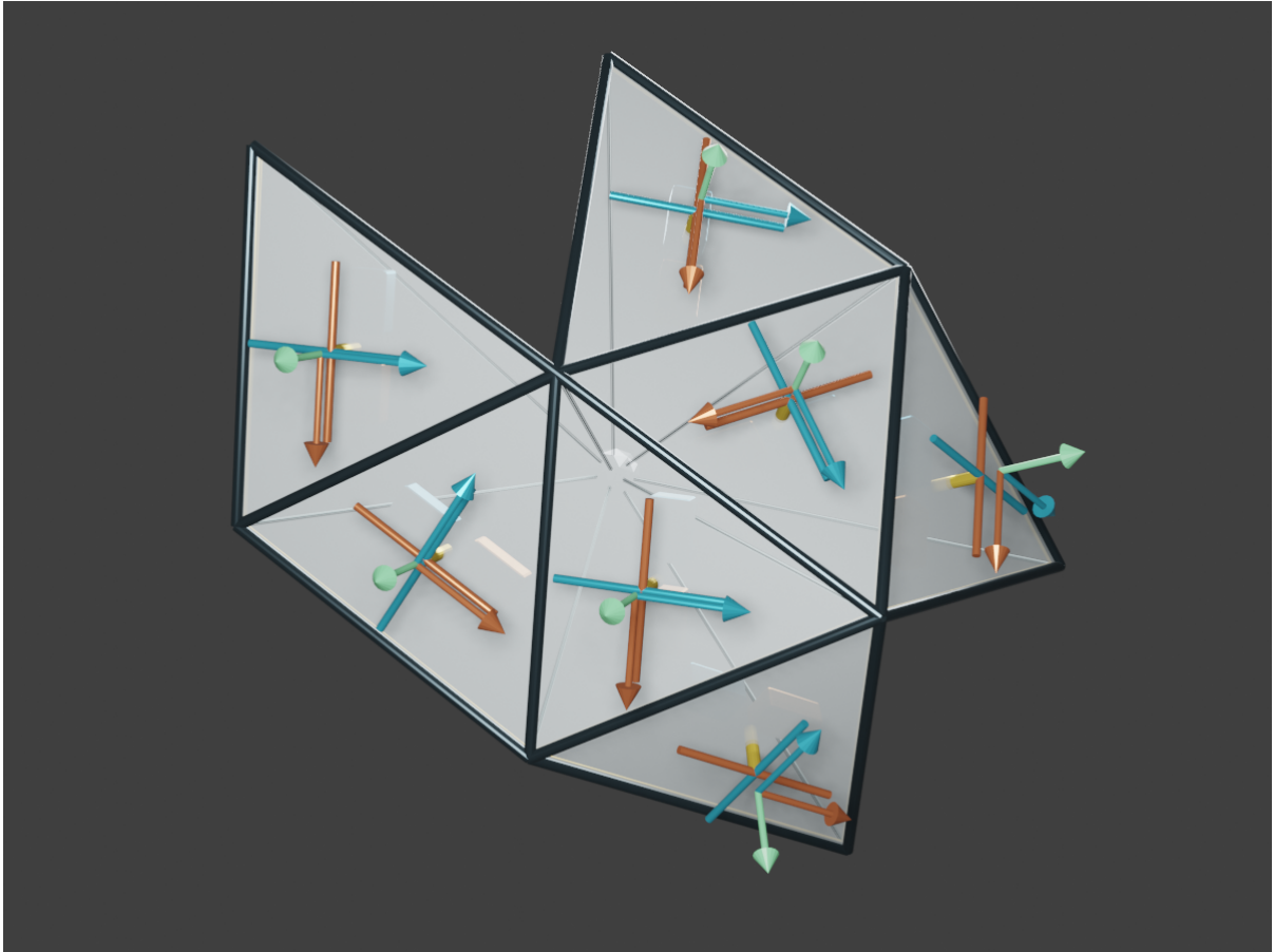
Figure 3.1: Seven contiguous tetrahedral face cells. Orange and cyan arrows show the local tangent basis, green arrows show outward normals, black rails show external structural seams, and the transparent lateral triangles converge to the common bonding hub / Sete células tetraédricas contíguas. As setas laranja e ciano mostram a base tangente local, as verdes mostram as normais externas, os trilhos pretos mostram as juntas estruturais externas e os triângulos laterais transparentes convergem ao hub comum de equipotencialização.
