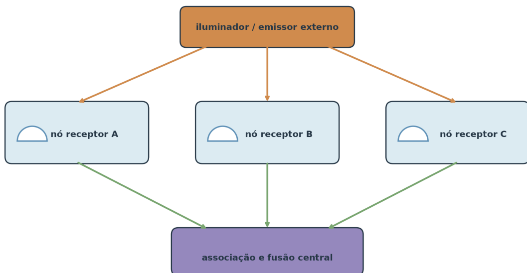
Figura 1 – Arquitetura distribuída de sensoriamento: o polígono superior representa um iluminador ou emissor, os três domos são nós receptores independentes, os caminhos verdes transportam observações calibradas e o bloco roxo inferior representa a fusão central.
