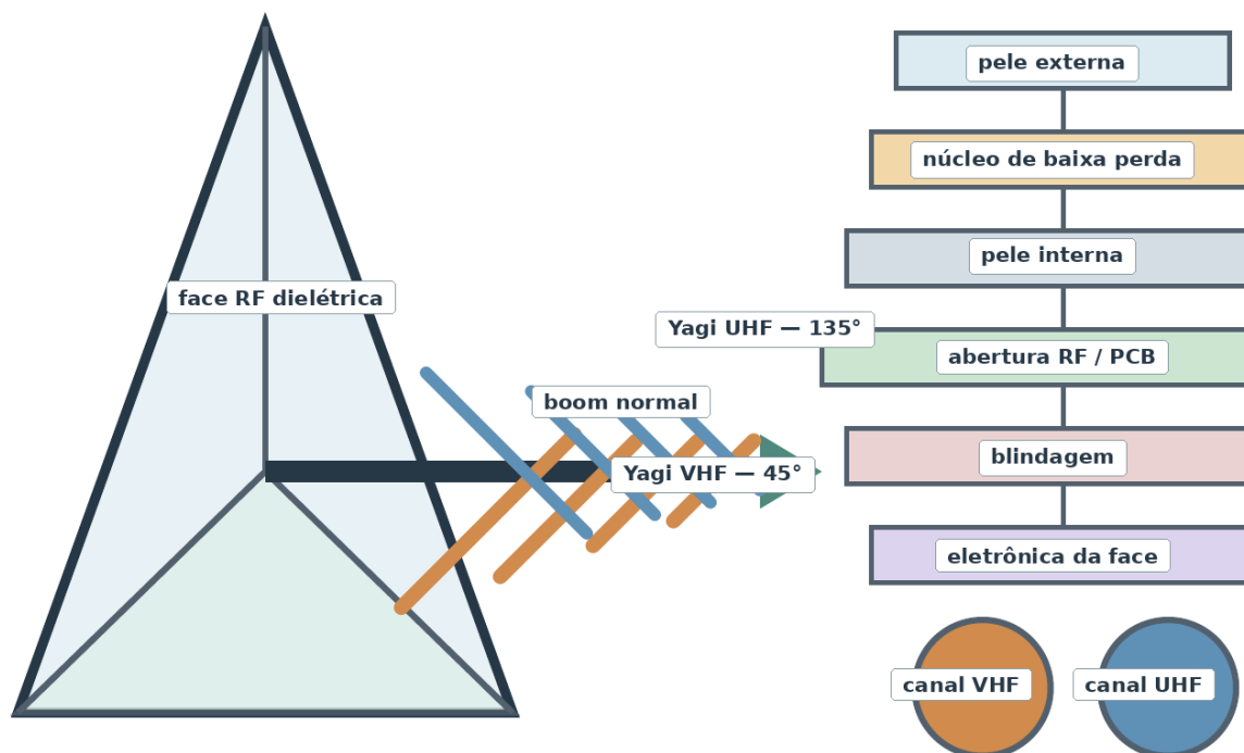
Figura 3 – Montagem de face. O boom escuro segue a normal externa desde o ápice interno e atravessa o centro da abertura triangular de dois metros; os elementos laranja e azul são mutuamente ortogonais e girados conjuntamente em 45^\circ ao redor dessa normal. As placas coloridas à direita representam a pilha de materiais e eletrônica.
