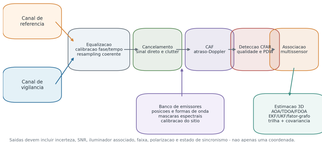
Figure 7.2: Multistatic passive processing / Processamento passivo multiestático.
