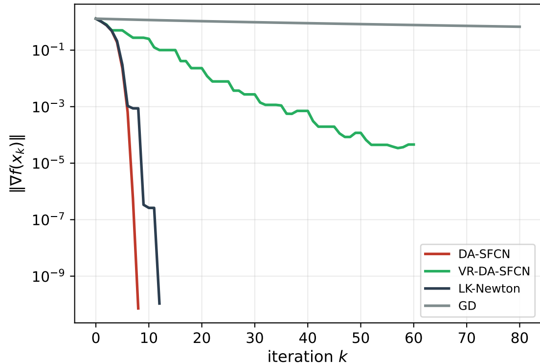
Finite-sum nonconvex quadratics
