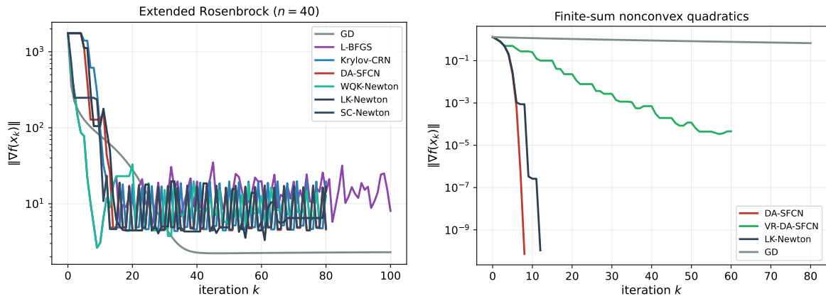
شكل 2: مجموع منتهٍ من التربيعيات وروزنبروك الممدّد.
