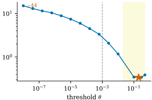
a9a (LIBSVM, real)
