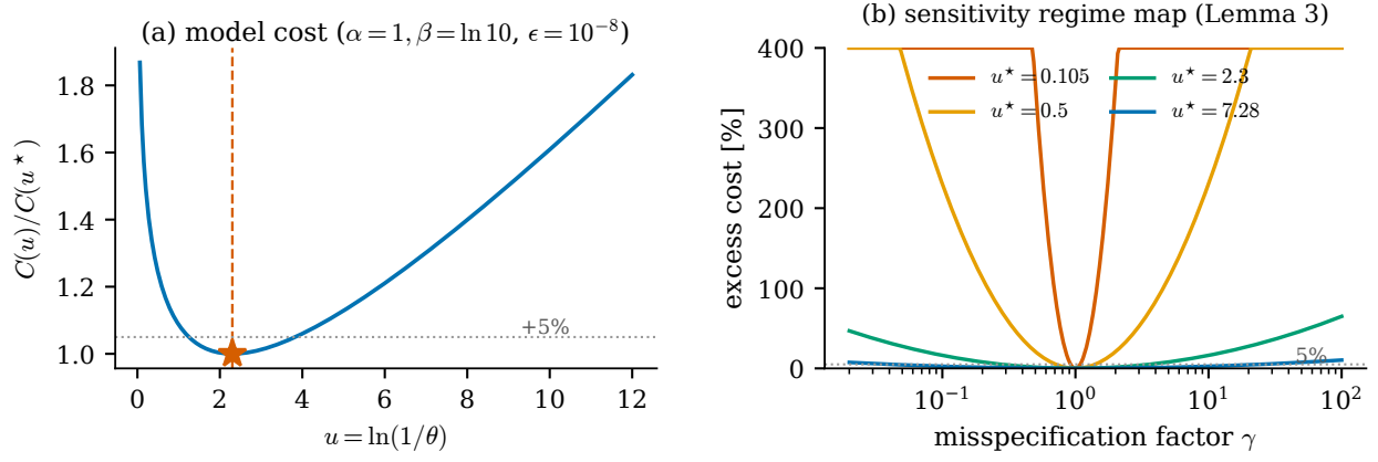
شكل 1: يسار: كلفة النموذج (2) ممتدة؛ الوعاء مسطح فعلاً داخل عامل عشرة من u^* . يمين: زيادة الكلفة لخطأ \gamma لعدة قيم u^* ؛ ينهار التسطح مع \theta^* \rightarrow 1 .
