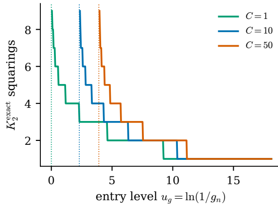
شكل 2: عدد الذيل الدقيق (نظرية 3b) مقابل مستوى الدخل لنسب انحاء C \in \{1, 10, 50\} . الخطوط المنقطعة هي البوابات \ln C : الاقتراب منها من أعلى يفجر عدد المربعات --- ثابت الحوض الخفي في النموذج مكشوفاً.
