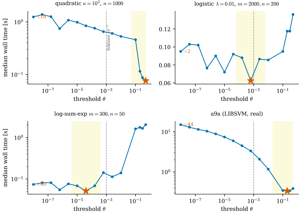
شكل 3: مسح E7 (وسيط الزمن مقابل \theta ; النجمة = الأمثل؛ الشريط \pm = عامل عشرة حوله؛ المنقط = البداية 10^{-3} ). لاحظ تغيّر الشكل بالعادة: متراجع رتبياً (التربيعي و a9a)، وأدنى داخلي مسطح حقاً (اللوغستي)، ومسطح يساراً/كارثي يميناً (log-sum-exp).
