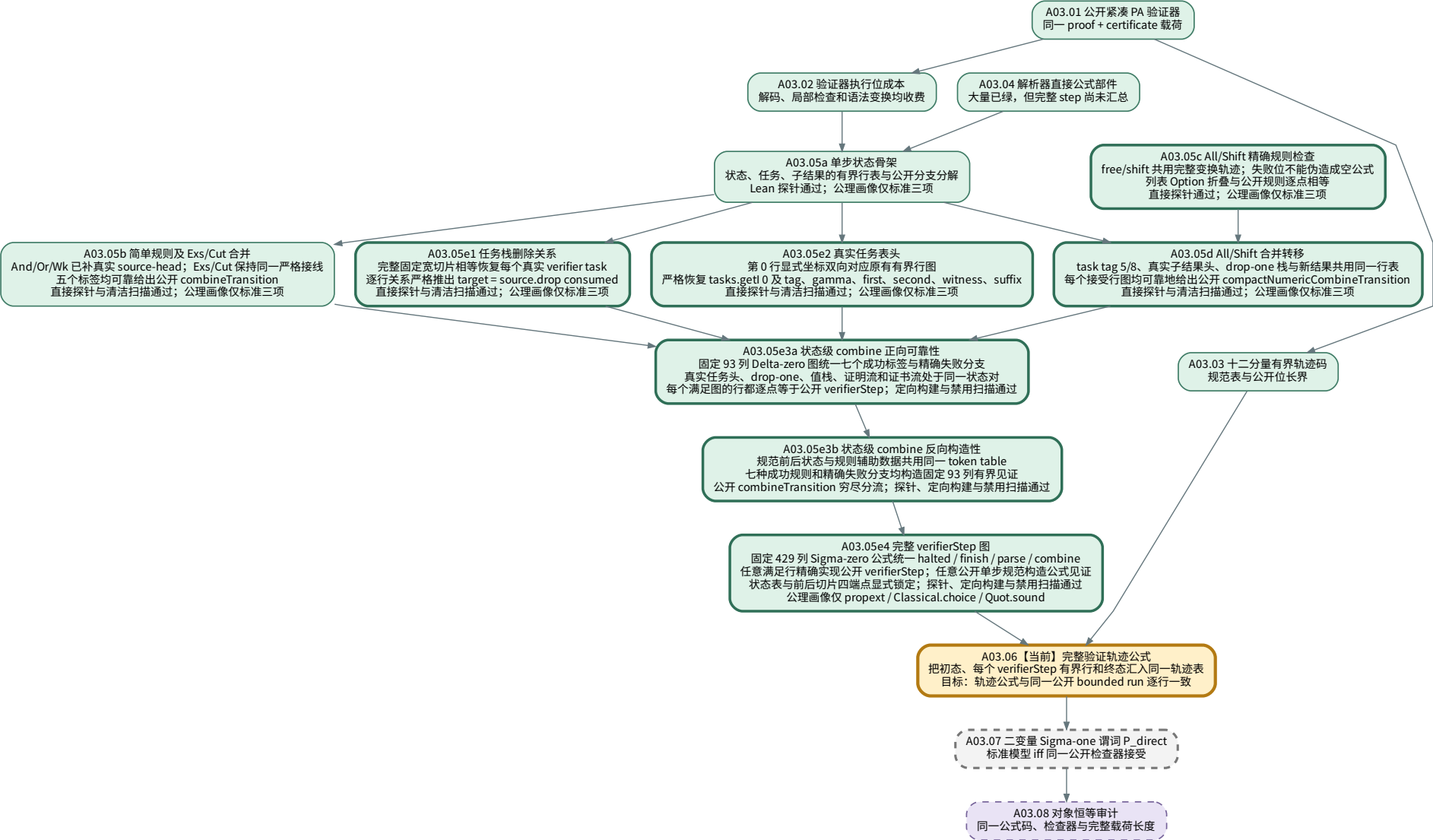
附图 03：验证器步骤与 P_direct
