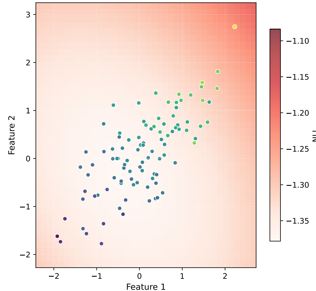
Cold VI Cold ( T=0.8 )
