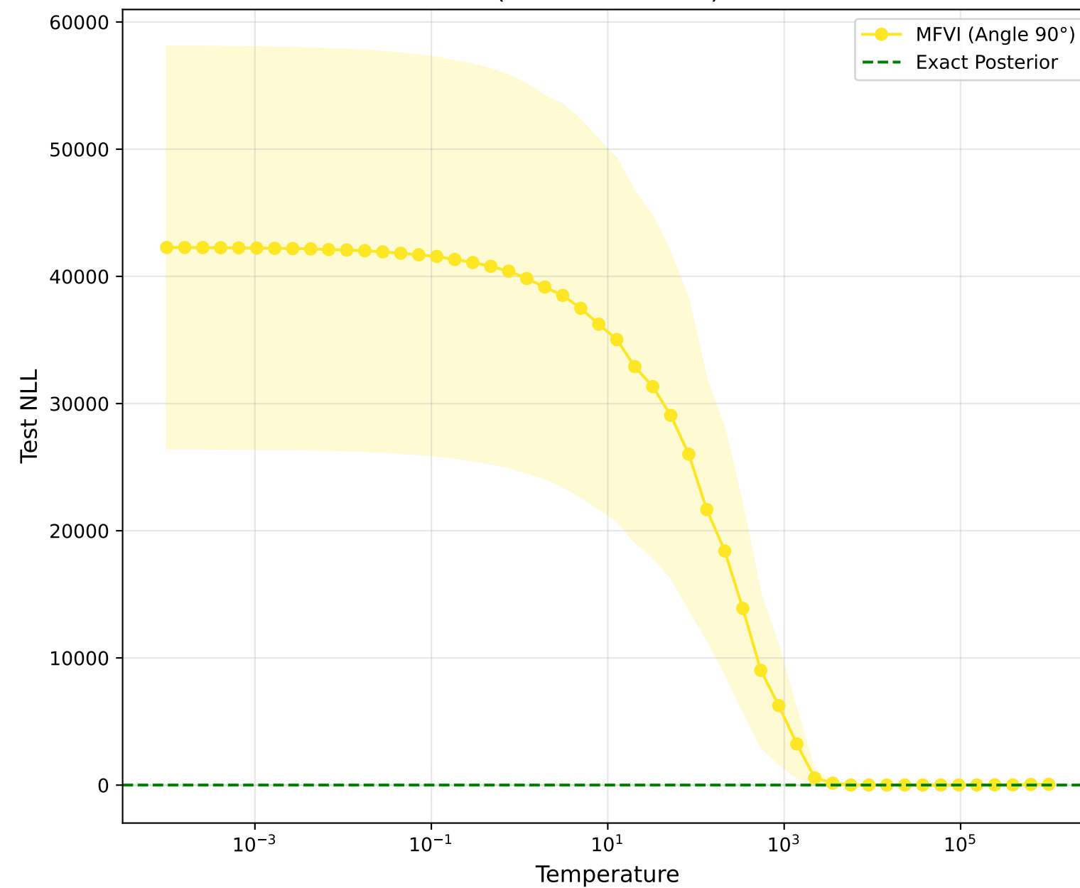
Weight Space Posterior (Run 0, 2SD)
