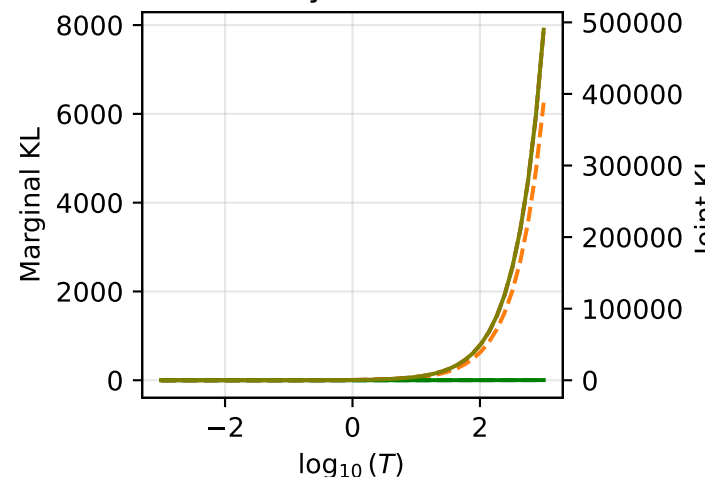
kin8nm
