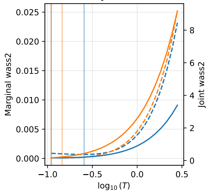
kin8nm
