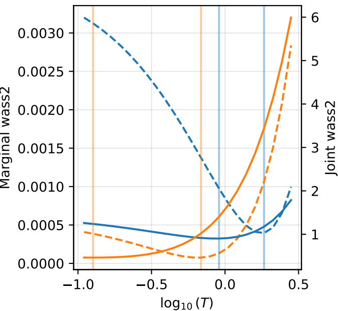
kin8nm
