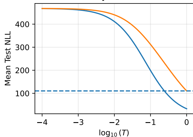
kin8nm
