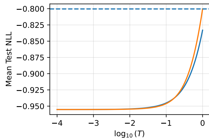
kin8nm
