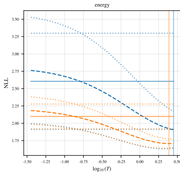
basis: rbf | NLL
