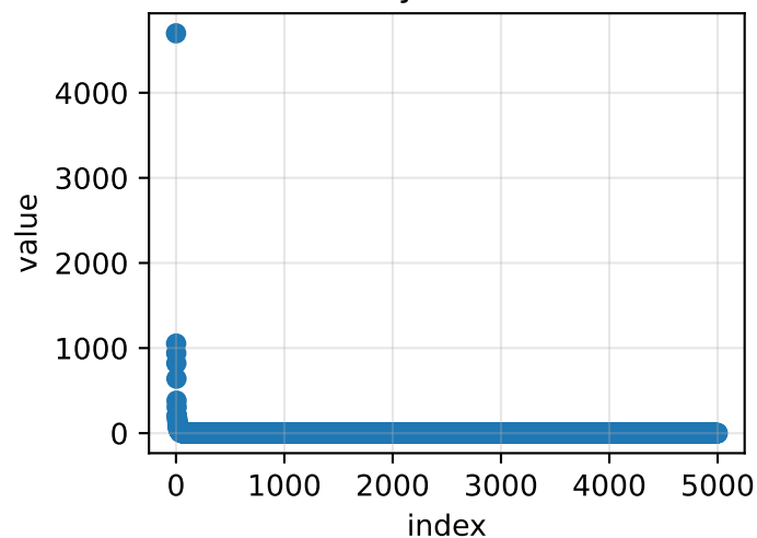
kin8nm
