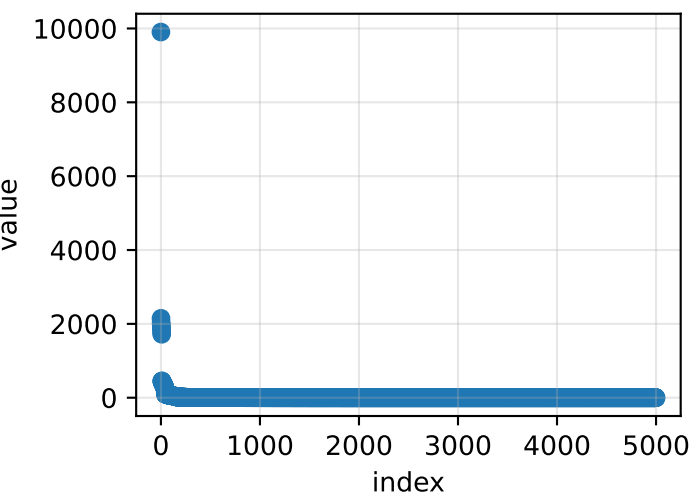
kin8nm
