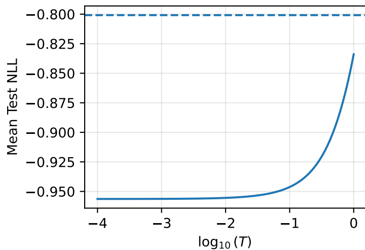
kin8nm
