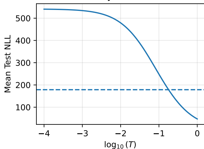
kin8nm
