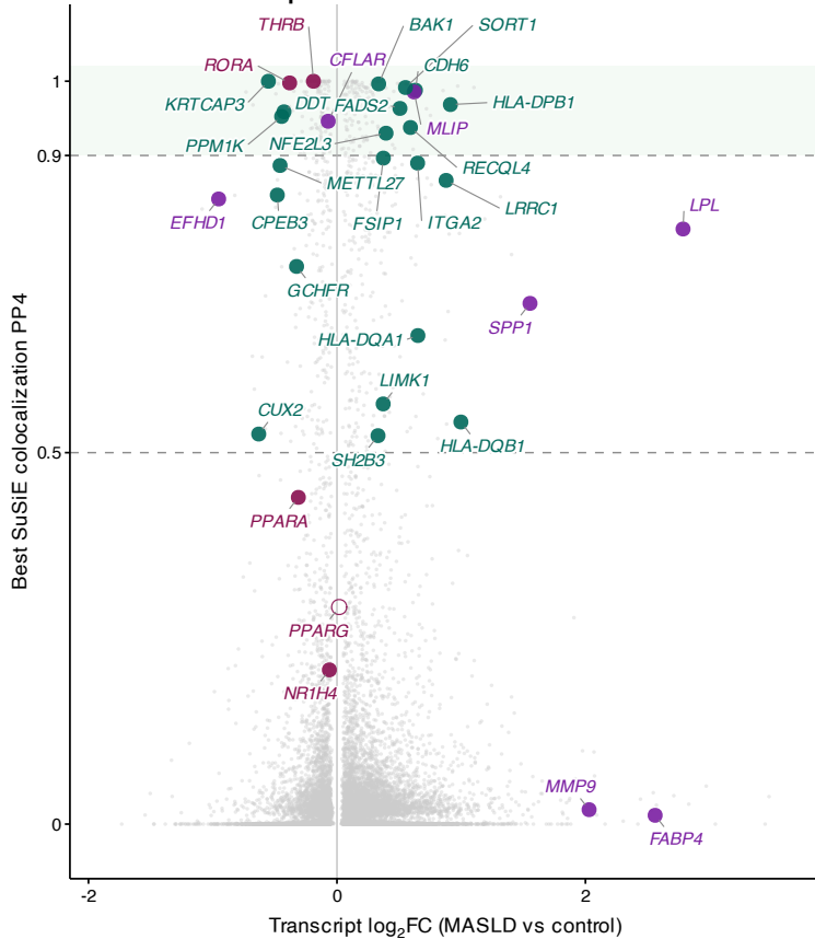
COLOC vs. RNA-seq DEG
