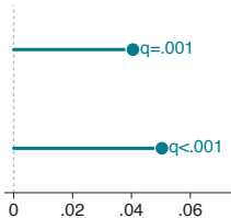
Stromal ECM
