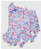
Stromal ECM
