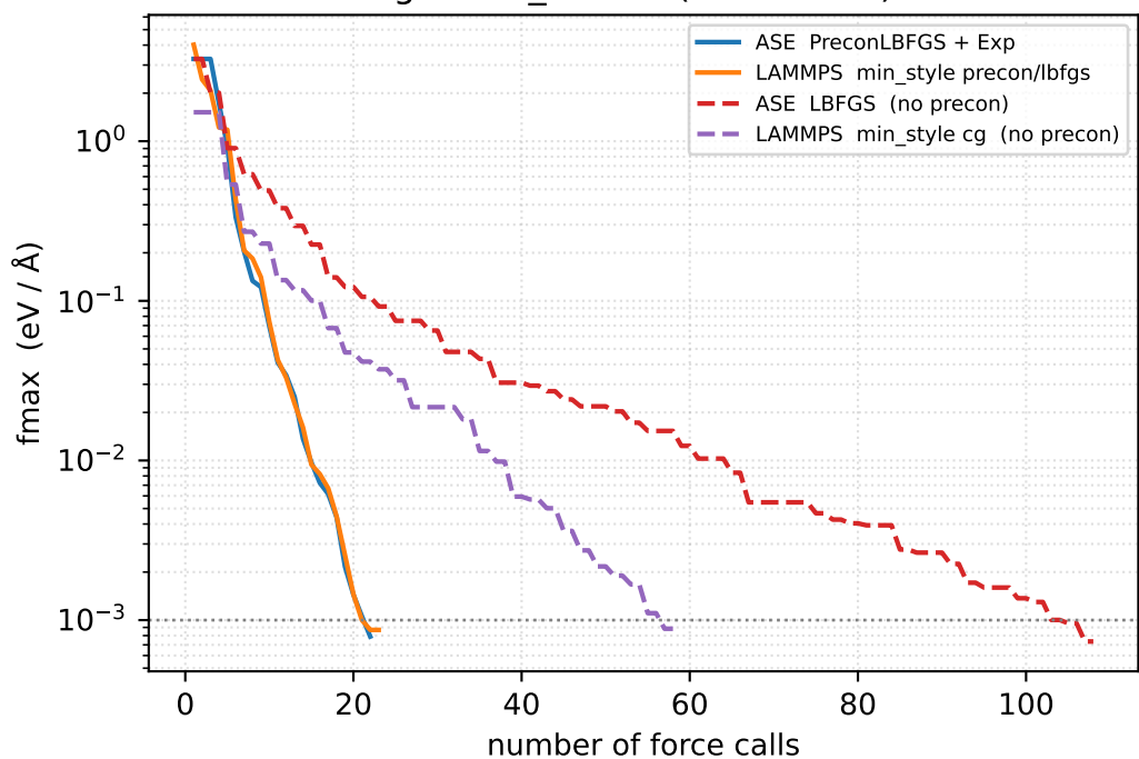
gamma_Al2O3 (106 atoms)
