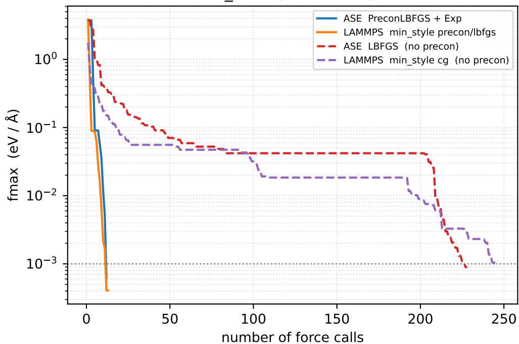
gamma_Al2O3 (106 atoms)
