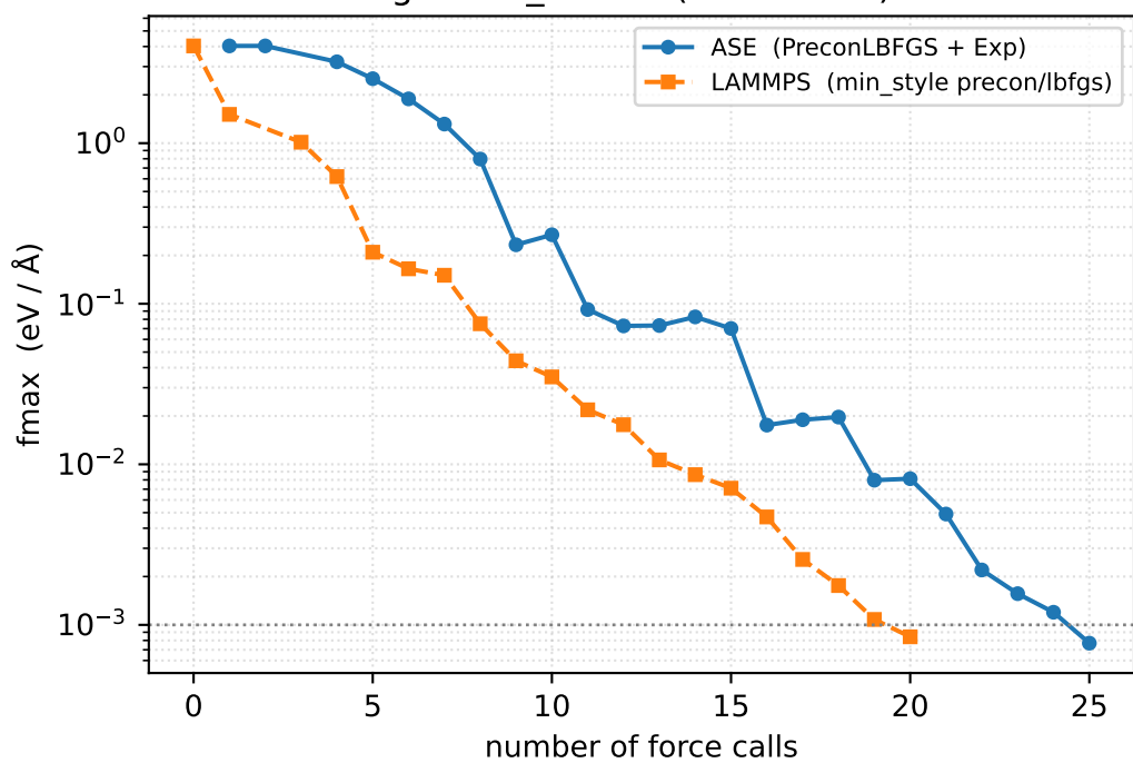
gamma_Al2O3 (106 atoms)
