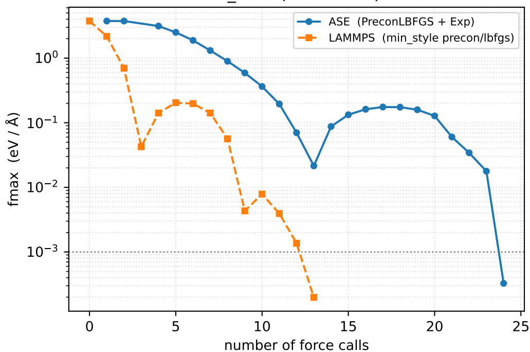
gamma_Al2O3 (106 atoms)
