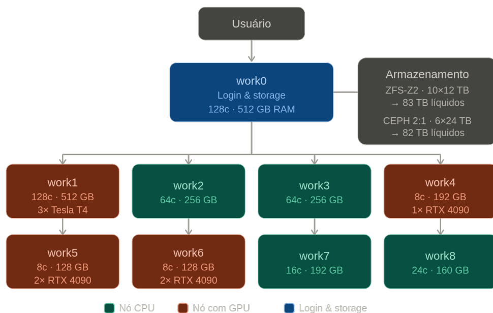
Figura 1: Arquitetura simplificada do Cluster Heisenberg.
