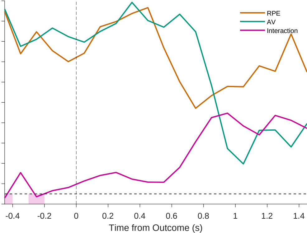
2-way ANOVA p-values
