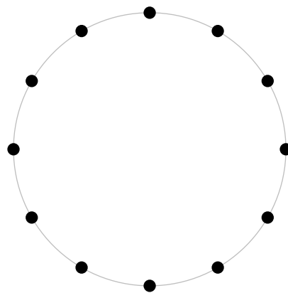
hop 6
