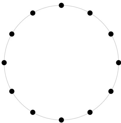
hop 5
