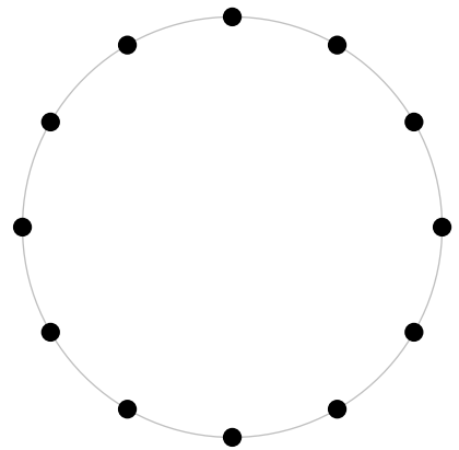
hop 4
