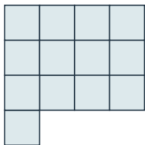
13 tiles: rows 4,4,4,1; P = 16
