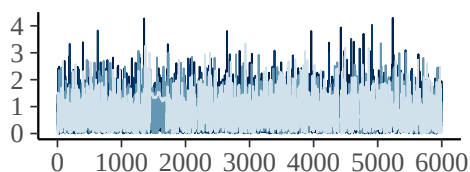
sds_stime_hours_1
