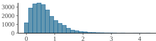
sds_stime_hours_1
