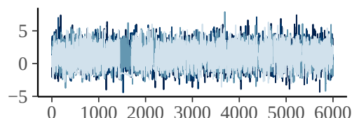
bs_stime_hours_1
