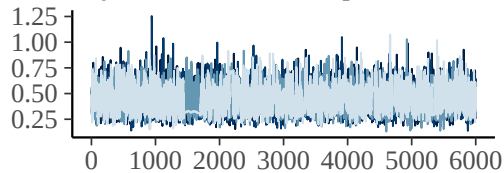
udy_id:arm:outcome_specific__Inte
