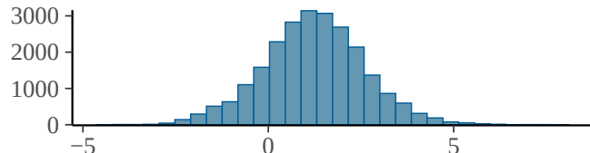
bs_stime_hours_1
