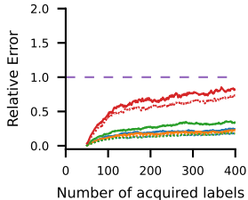
7B-zero
