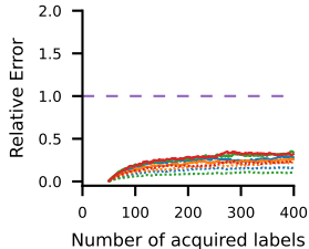
70B-zero
