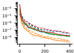
MSE-estimation error
