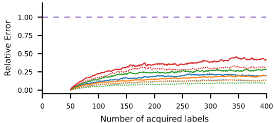
Gemma3-4b-zero
