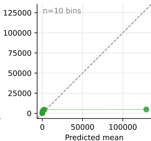
GLMM-Oracle
