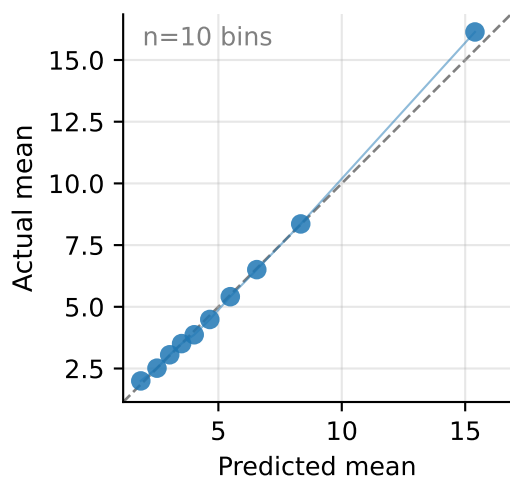
SaaS (ZI-Gamma)
