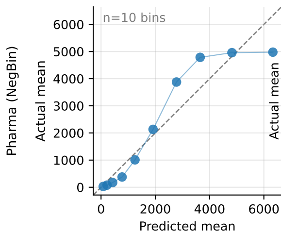
TreeMMM
