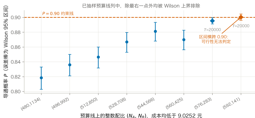
图 10 预算线上抽样审计： P 的点估计与 Wilson 区间
