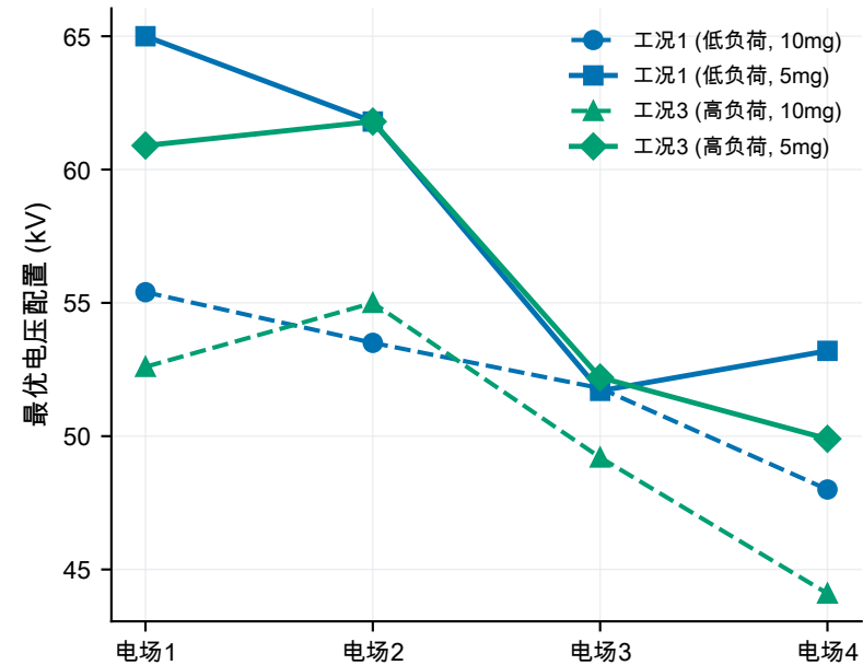
(a) 代表工况四电场电压阶梯分布
