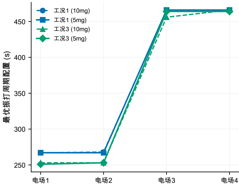
(b) 代表工况四电场振打周期分布
