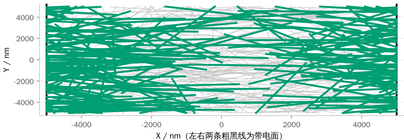
组3：354 根介质 A (535 个碎片)，截面 10000×10000 nm —— 导通
