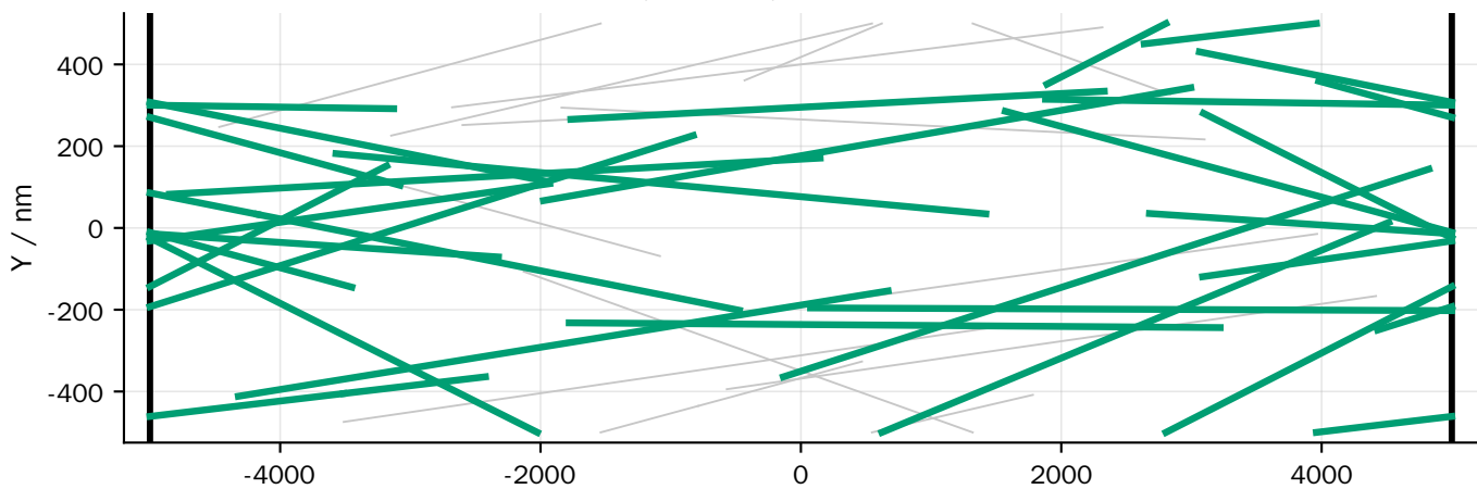
组3：354 根介质 A（535 个碎片），截面 10000×10000 nm —— 导通
