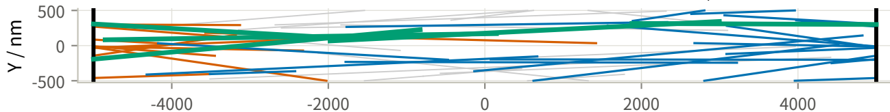
组3: 354根介质 A (535个碎片), 截面 10000 \times 10000 \text{ nm} —— 导通 (贯通团簇 17/535个碎片)
