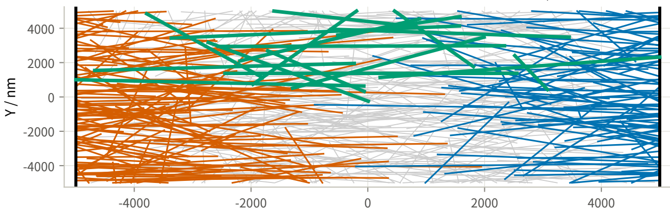
组3: 354根介质 A (535个碎片), 截面 10000 \times 10000 \text{ nm} —— 导通 (贯通团簇 17/535个碎片)
