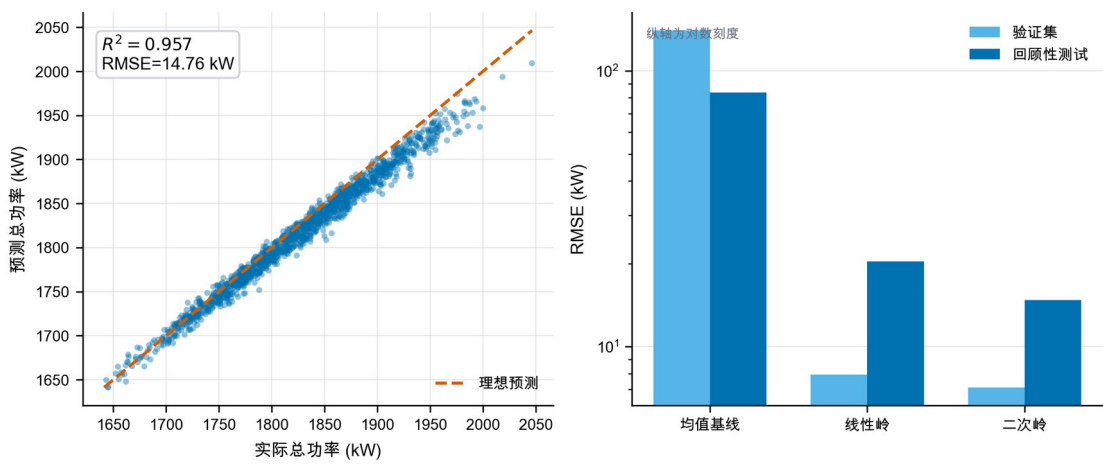
图 8 二次岭在回顾性测试上保持较高一致性，并优于均值与线性基线。左图虚线为理想预测；右图 RMSE 采用对数纵轴，使三种模型的量级差异同时可见。
