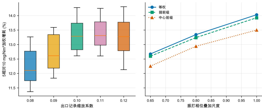
图 17 405 组灰箱参数组合情景的增耗分布。出口缩放与振打相位会系统改变增耗，中心点约 13.7%应与 11.37%~14.31%的灰箱参数组合情景范围一起解释。
