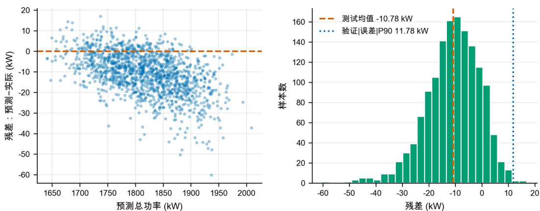
图9 回顾性测试残差诊断。平均偏差为-10.78 kW，高功率区负偏差有所扩大；验证绝对误差90%分位数 11.78 kW 被用作验证期误差附加量。上线前仍需用全新日期重新校准，不能把当前测试称为真正盲测。
