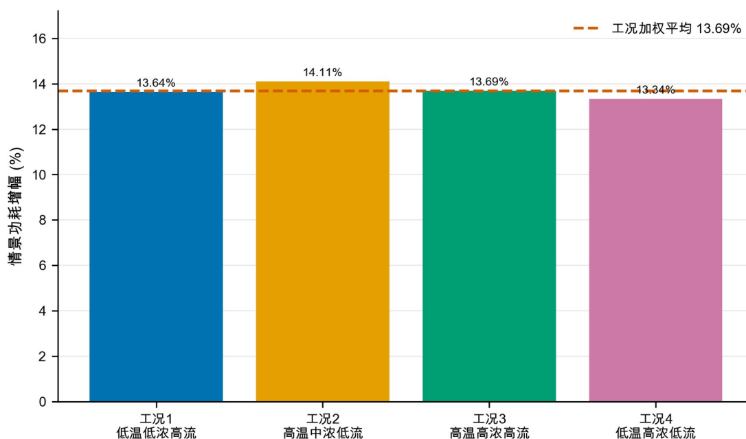
图 14 四工况从 10 收紧至 5 mg/Nm 3 的中心情景增耗。分工况为 13.34%~14.11%，工况加权点估计约 13.7%；该点值必须与灰箱参数组合情景范围同时报告。
