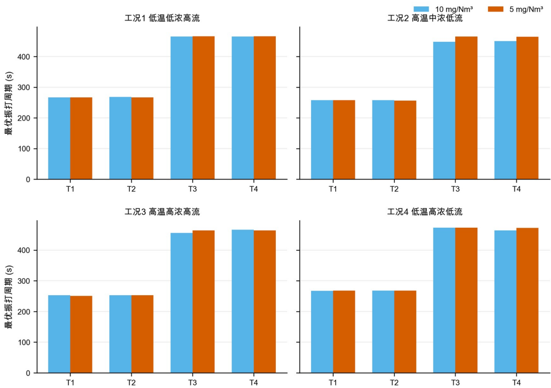
图 13 两档排放限值下的中心情景最佳采样振打周期。周期变化不像电压那样单向，而是在积灰损失与再飞扬峰值间重新平衡；前级短、后级长的顺序保持不变。
