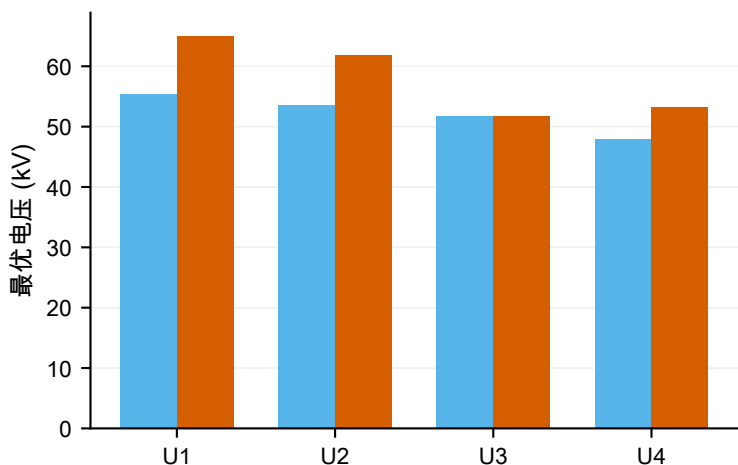
(a) 工况1 低温低浓高流
