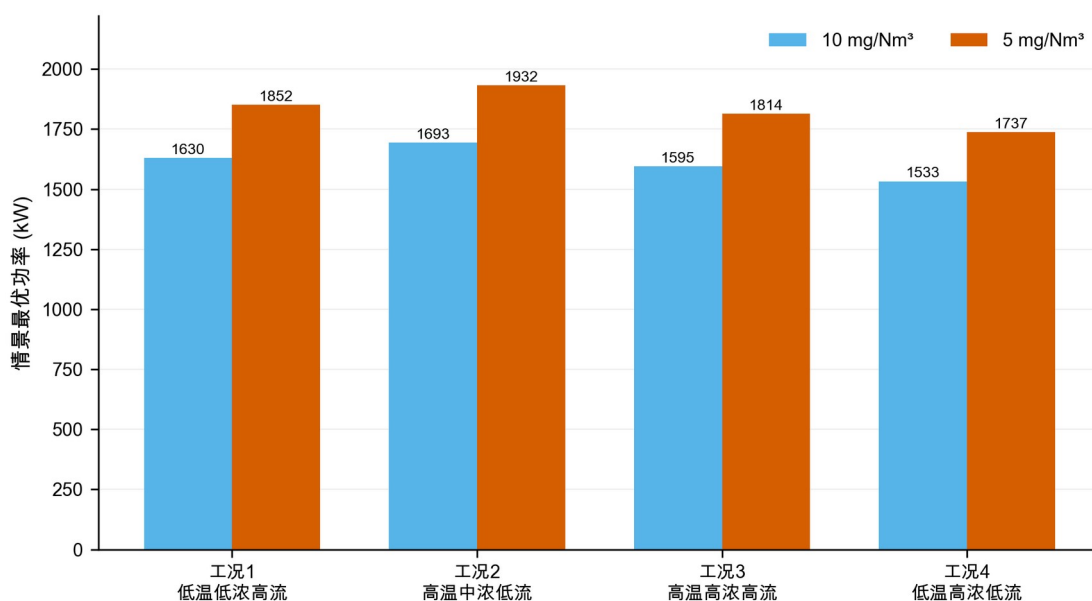
图 13 两档排放限值下的最佳采样功耗
