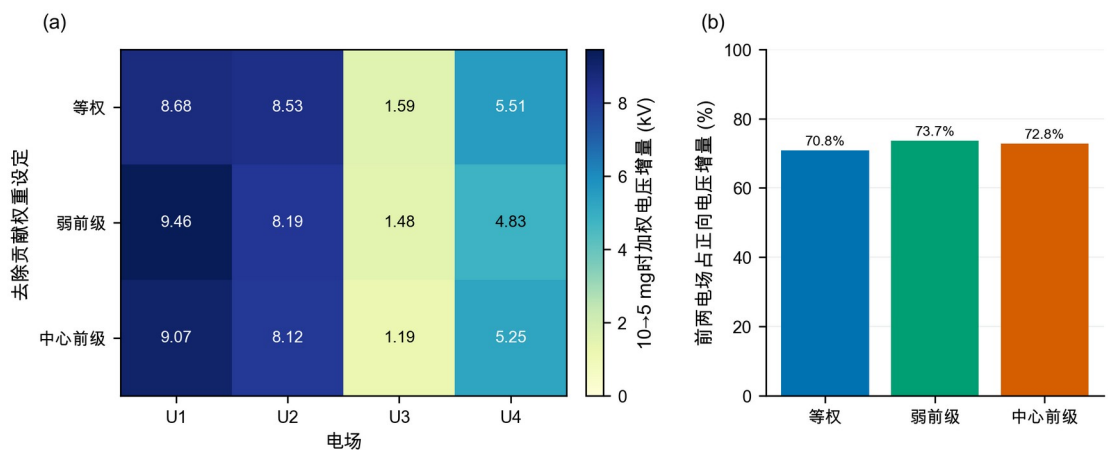
图 21 电场贡献权重消融结果
