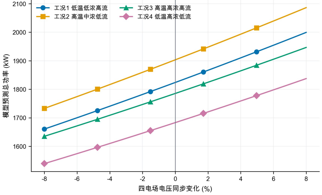
图 11 局部电压—功耗响应
