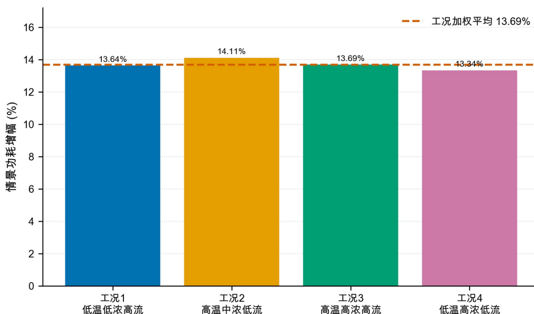
图 17 分工况增耗比较
