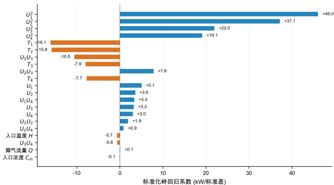
图9 二次岭功耗模型的标准化系数
