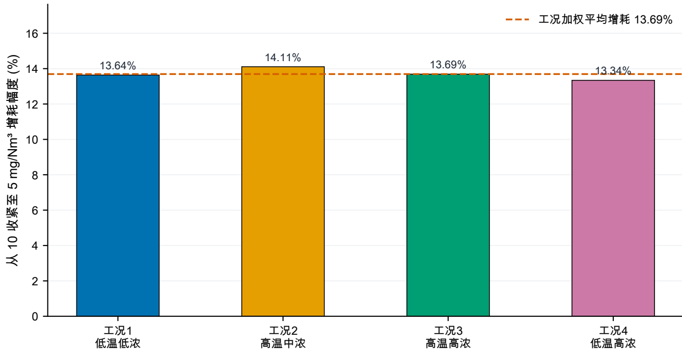
四类工况由 10 mg/Nm 3 收紧至 5 mg/Nm 3 的增耗分布
