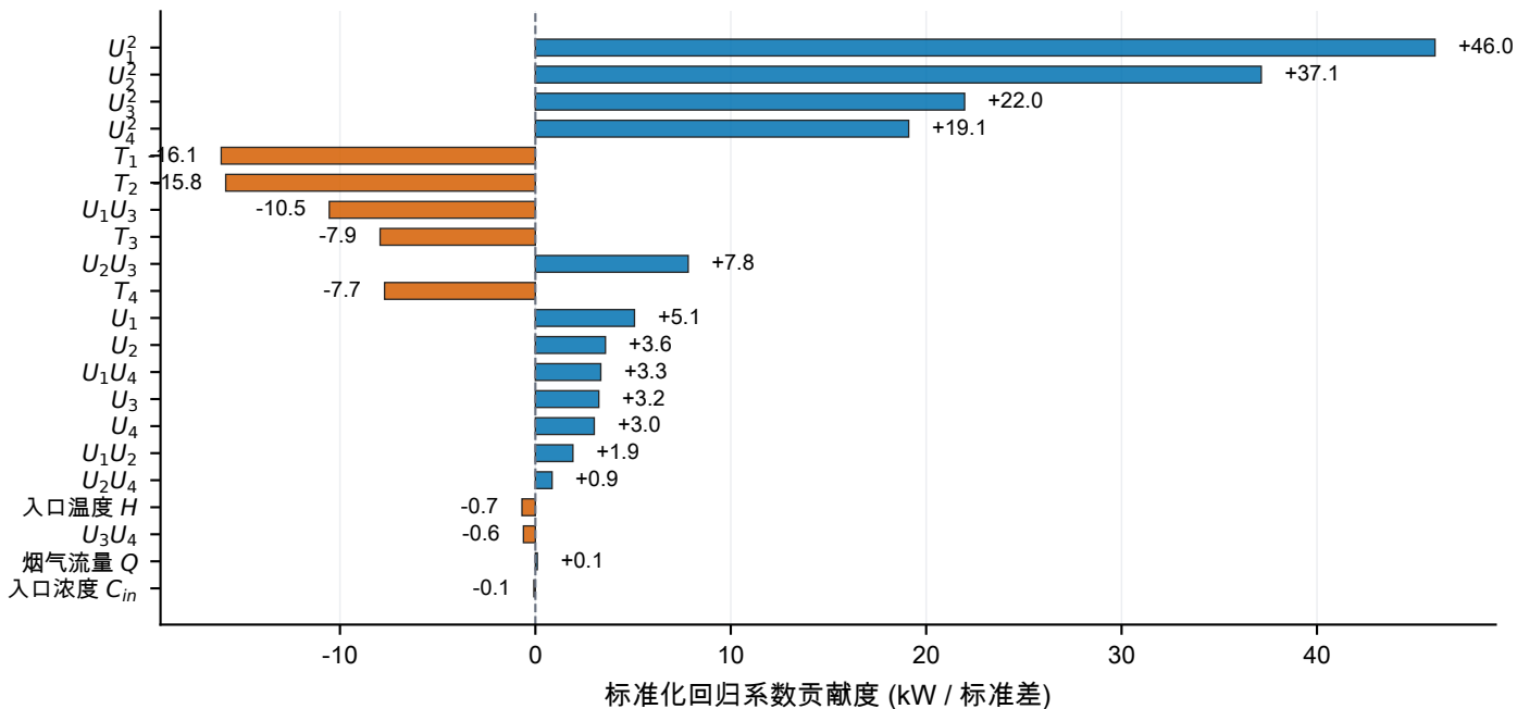
二次岭功耗模型各特征变量标准化贡献度排序
