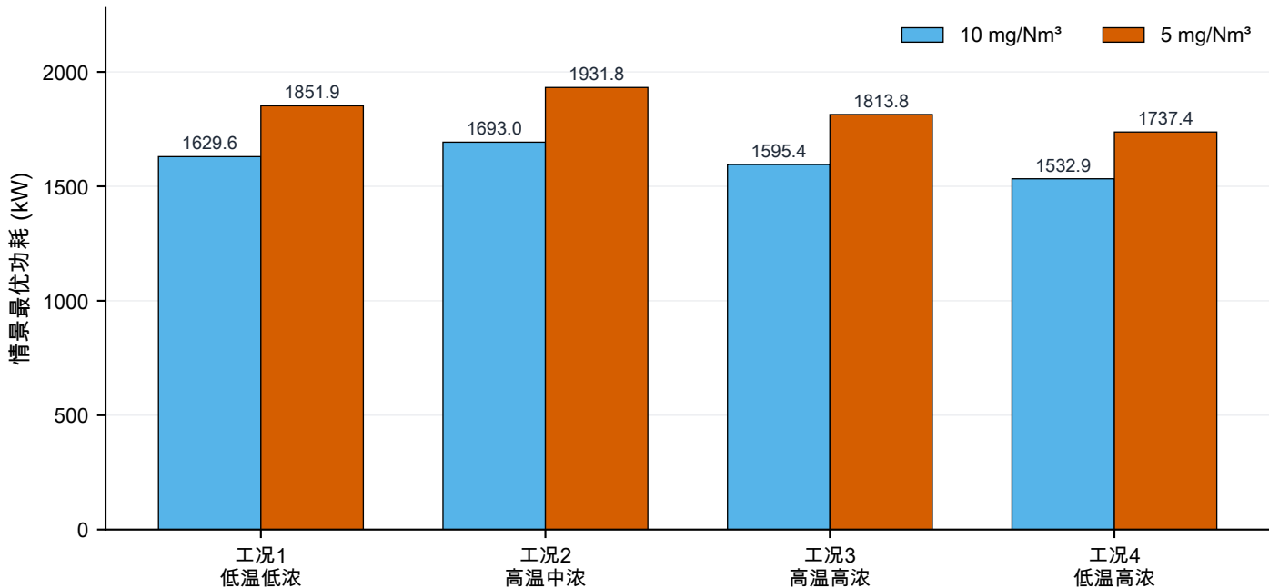
四工况在 10 和 5 mg/Nm 3 排放约束下的情景最优功耗对比
