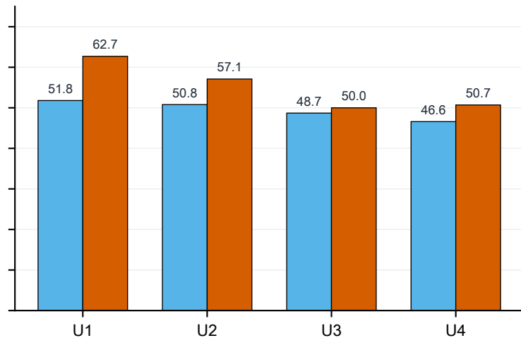
工况 4 最优电压配置 (kV)
