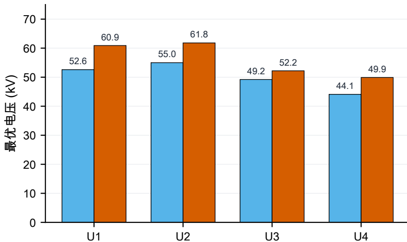
工况 3 最优电压配置 (kV)
