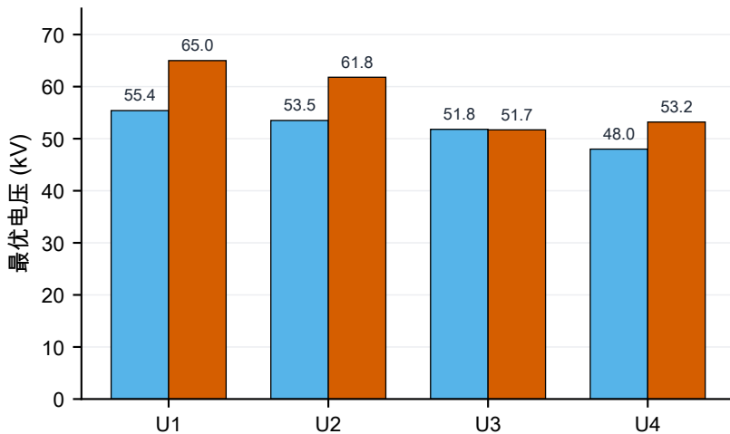
工况 1 最优电压配置 (kV)
