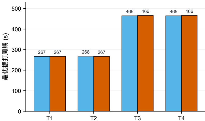
工况 1 最优振打周期配置 (s)
