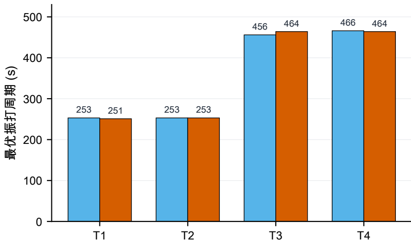
工况 3 最优振打周期配置 (s)
