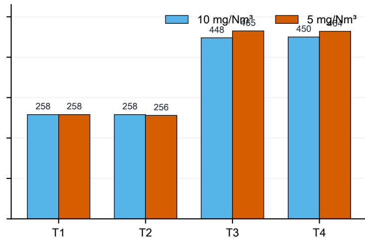
工况 2 最优振打周期配置 (s)
