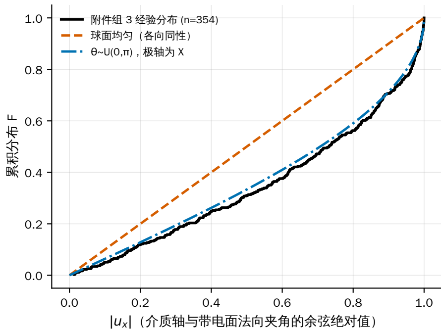
KS 检验：各向同性 p=6.7e-19 ，极角均匀 p=0.73
