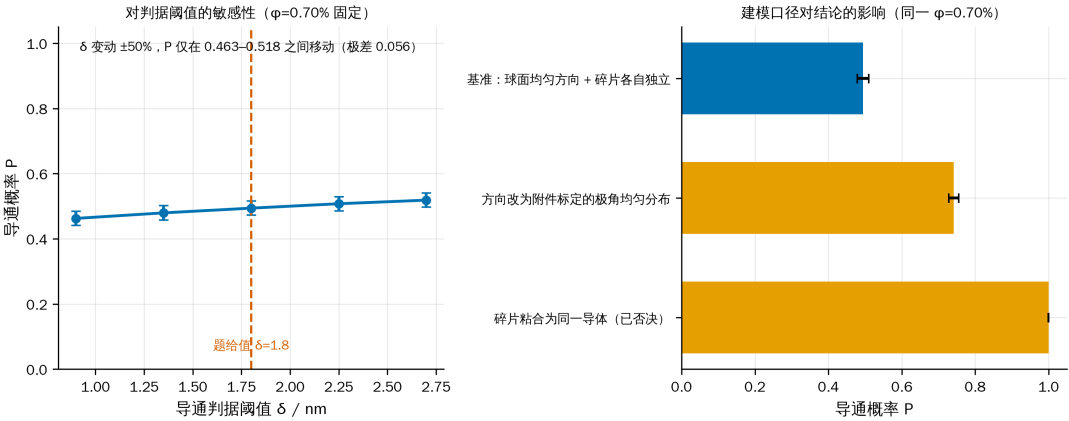
图 8 导通概率对判据阈值与建模口径的敏感性
