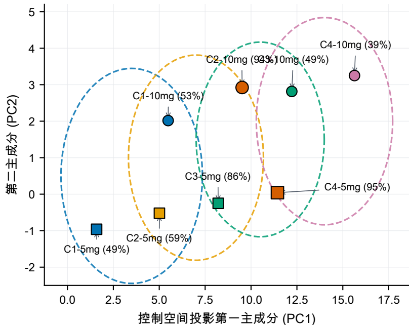
(a) 推荐解在马氏距离椭圆域内的投影
