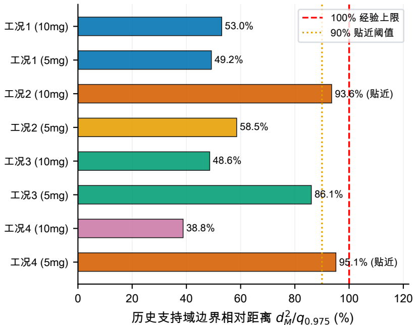
(b) 推荐解的支持域边界贴近度
