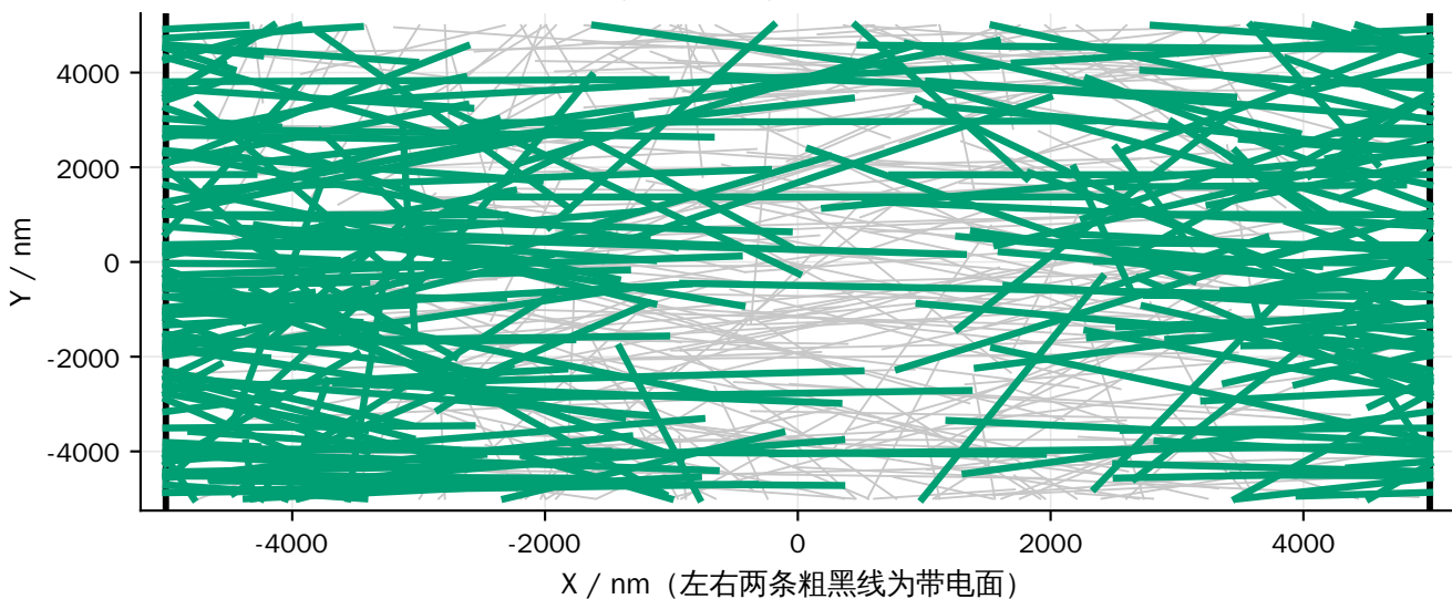
组3：354 根介质 A（535 个碎片），截面 10000×10000 nm —— 导通
