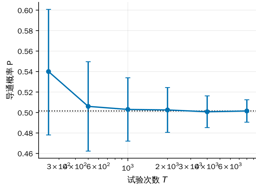
估计值随样本量的稳定过程 ( \varphi=0.70\% )
