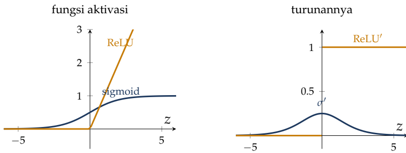
Gambar 12.2: Sigmoid versus ReLU. Kiri: bentuk fungsinya. Kanan: turunannya. Turunan sigmoid (biru) mengecil ke nol di kedua ekor (sumber vanishing gradient ), sedangkan turunan ReLU (amber) tetap 1 untuk semua masukan positif, sehingga gradien mengalir utuh.
