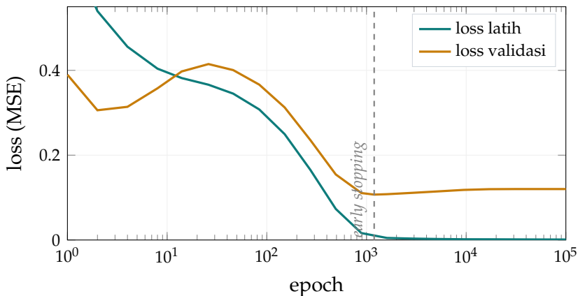
Gambar 12.1: Overfitting nyata. Loss latih (teal) terus turun, tetapi loss validasi (amber) berbalik naik setelah titik tertentu. Garis putus-putus menandai saat loss validasi terendah, yaitu tempat ideal untuk berhenti.
