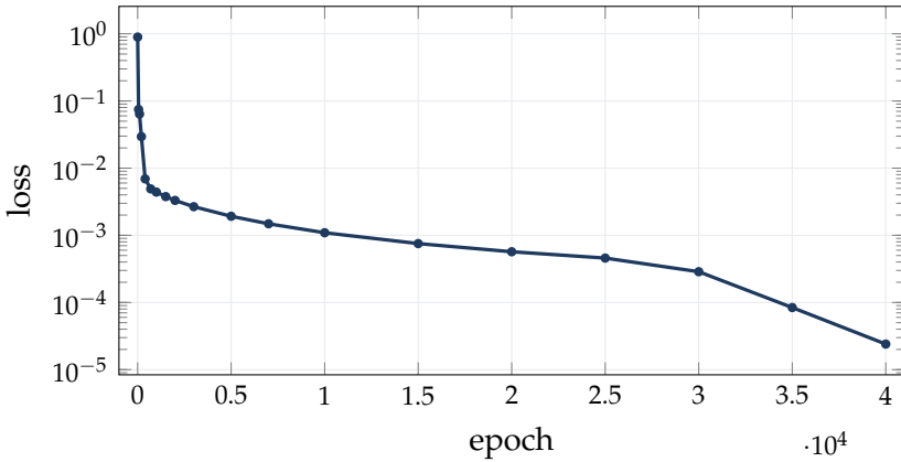
Gambar 6.1: Loss selama pelatihan (skala log). Dari \approx 0,89 menuju \approx 0,00002 . Penurunan curam di ratusan epoch pertama lalu melandai, sebuah pola yang khas pada gradient descent .
