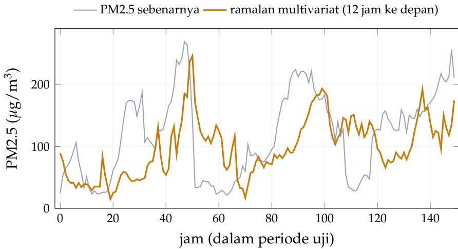
Gambar 11.1: Ramalan polusi multivariat 12 jam ke depan (amber) versus nilai sebenarnya (biru) untuk 150 jam pertama periode uji. Jaringan menangkap pola besar naik-turunnya polusi, meski melewati sebagian puncak paling tajam yang sulit diramal sejauh dua belas jam.
