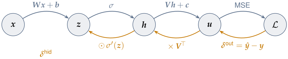
Gambar 4.1: Dua arah aliran. Di atas (biru), forward pass membawa nilai dari x ke \mathcal{L} . Di bawah (amber), backward pass membawa gradien mundur dari \mathcal{L} : mulai dari \delta^{\text{out}} di u , dikalikan V^T untuk pindah ke ruang h , lalu dikali per-elemen \sigma'(z) menjadi \delta^{\text{hid}} di z .
